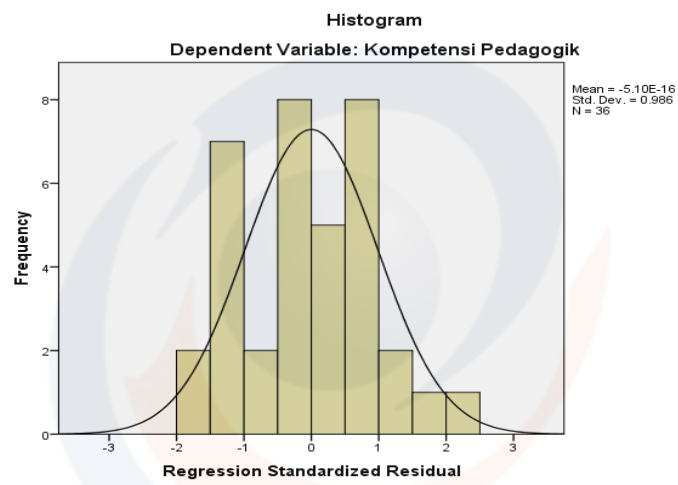
Gambar 5.1 Grafik Histogram Normalitas
