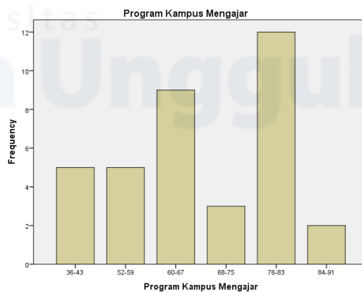
Gambar 4.1 Grafik Distribusi Frekuensi Program Kampus Mengajar
