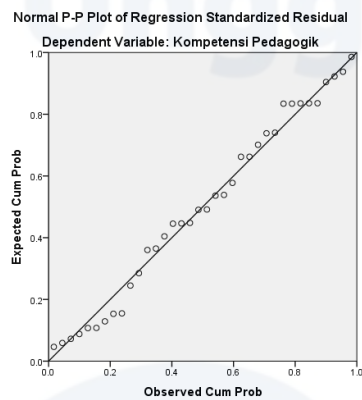
Gambar 5.2 Grafik Normal P.P Plot
