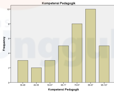
Gambar 4.2 Grafik Distribusi Frekuensi Kompetensi pedagogik
